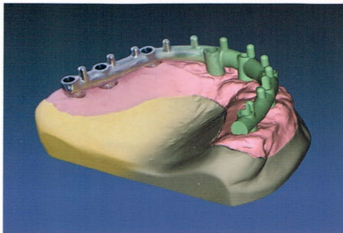
Diseño virtual y real de una barra híbrida.
